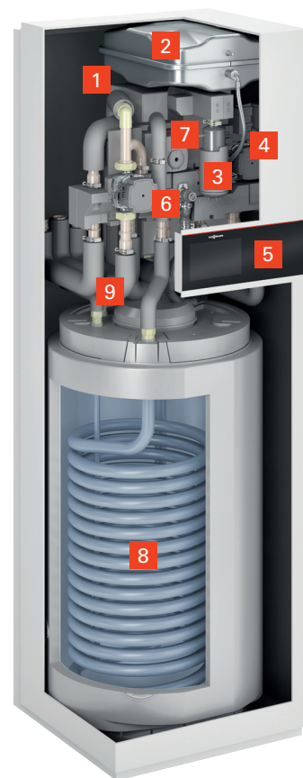
VITOCAL 252-A Avec deux circuits de chauffage/refroidissement
