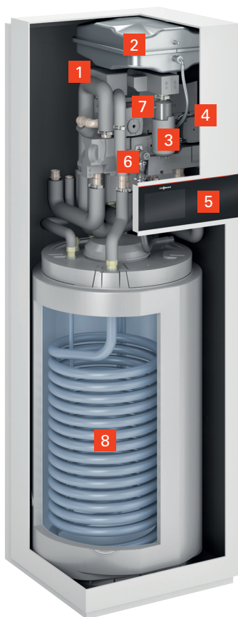
VITOCAL 252-A Avec un circuit de chauffage/refroidissement intégré
