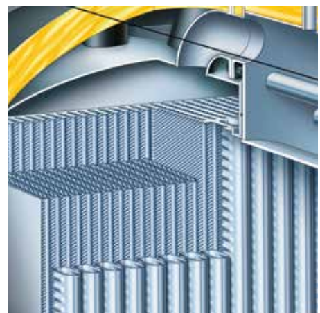
Inox-Crossal-verwarmingsoppervlak voor een zeer efficiënte warmteoverdracht en condensatiebenutting
