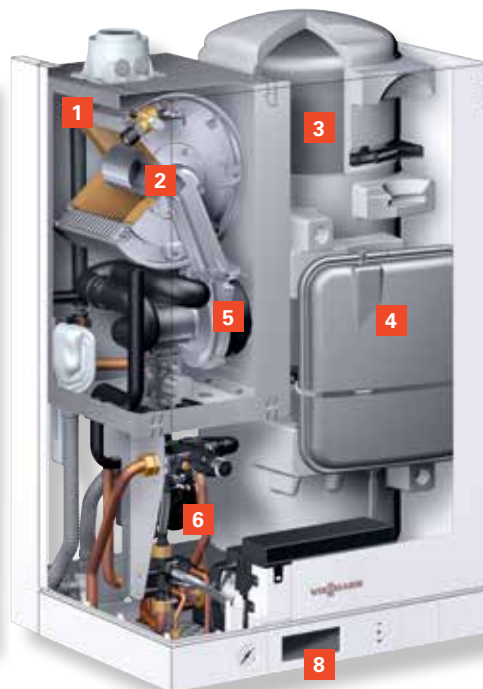
Vitodens 111-W
