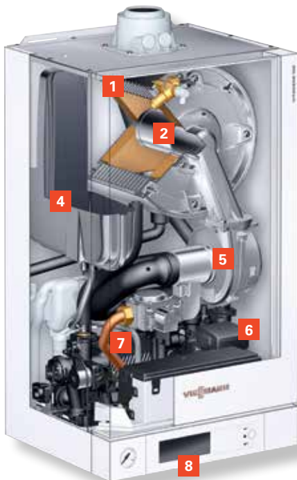
Vitodens 100-W (condenserende combiketel weergegeven)
